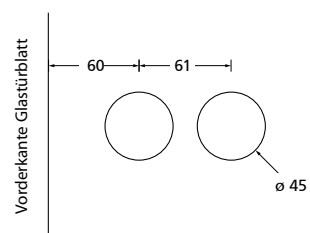
Bohrmaße Glastürschloss
